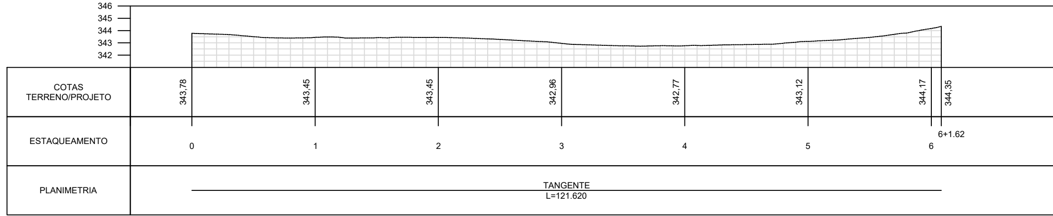
PERFIL ALINHAMENTO - RUA FREI DAMIÃO
