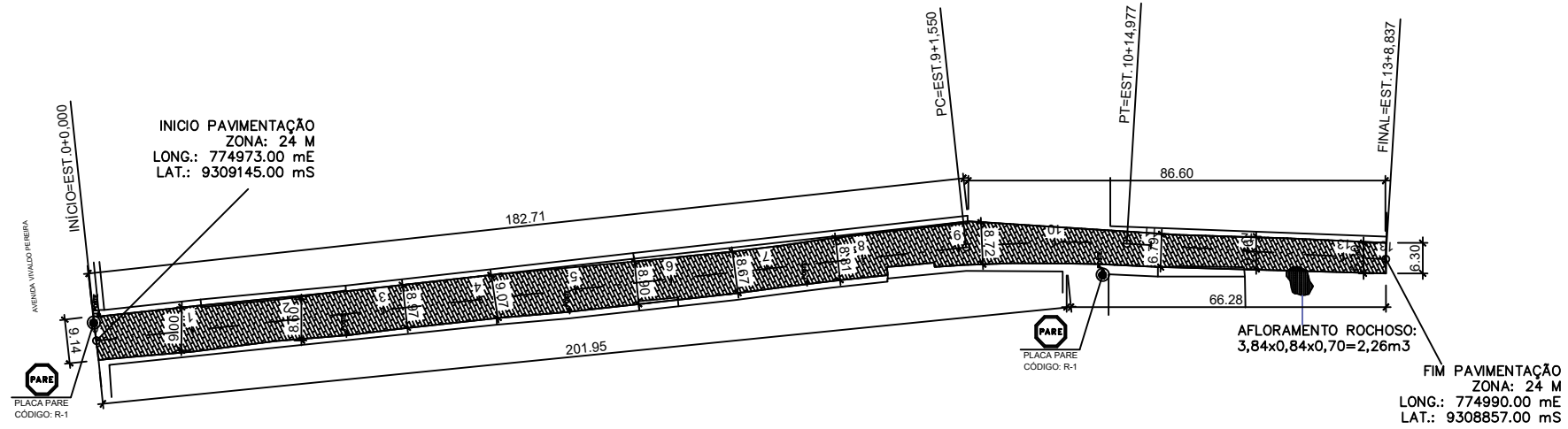
PLANTA BAIXA - RUA: CHICÓ CAZUA ESC: 1/500
