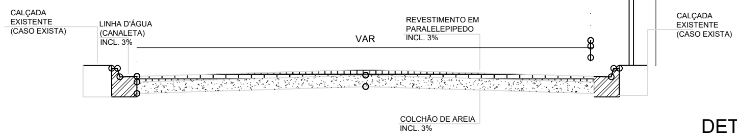
RUA: ANTONIO GOMES MELO SEM ESCALA
