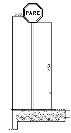
DETALHE DA PLACA DE SINALIZAÇÃO SEM ESCALA
