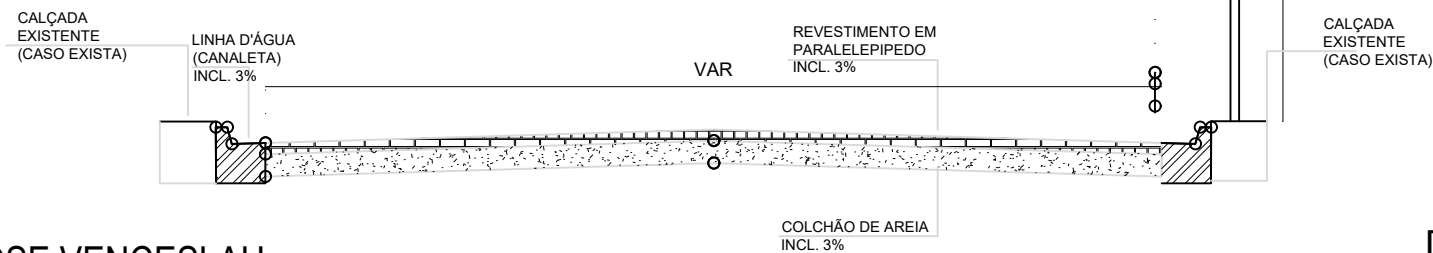
RUA: JOSE VENCESLAU SEM ESCALA
