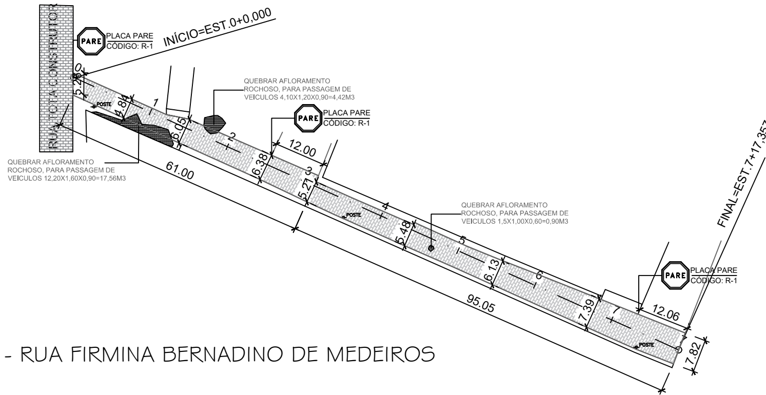
PLANTA DE LOCALIZAÇÃO - RUA FIRMINA BERNADINO DE MEDEIROS SEM ESCALA
