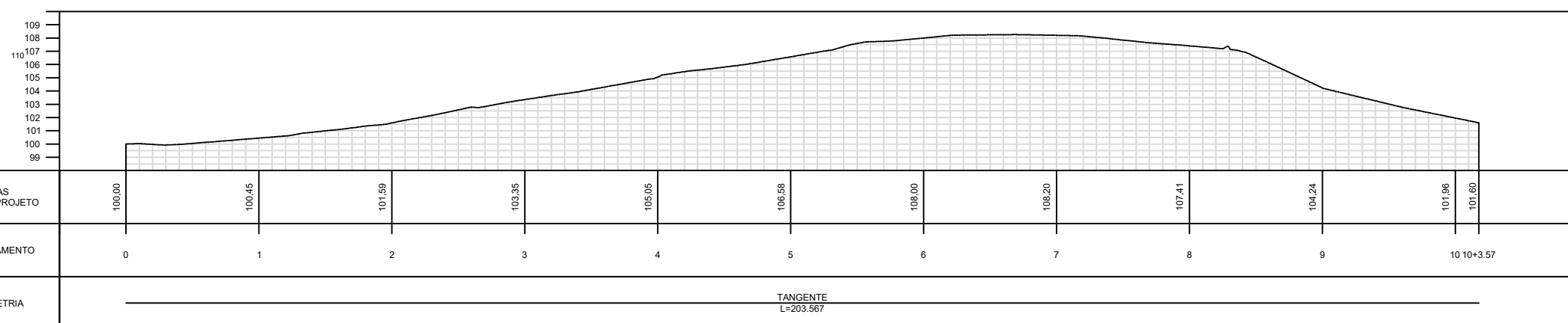
PERFIL RUA MIZAEI XAVIER GOMES
