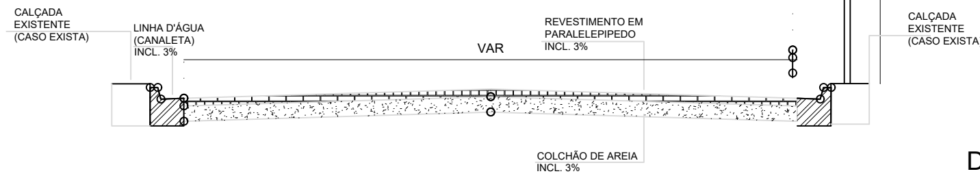
RUA: MIZAEI XAVIER SEM ESCALA
