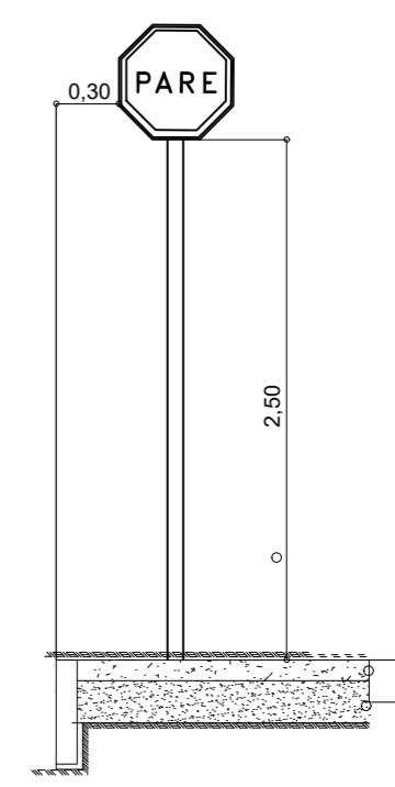
DETALHE DA PLACA DE SINALIZAÇÃO SEM ESCALA
